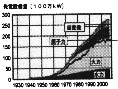
図7 発電設備容量と最大必要電力量の推移
